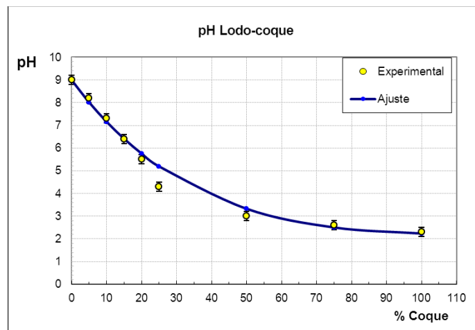
Figura 6. Potencial de hidrógeno en función de la concentración de coque en el lodo rojo una vez tratado a 1000 °C
