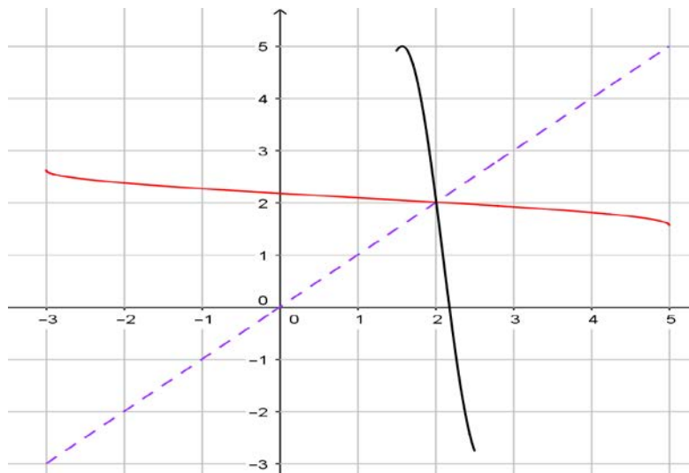
Figura 9. Representación gráfica en GeoGebra de la restricción de f y su inversa.
