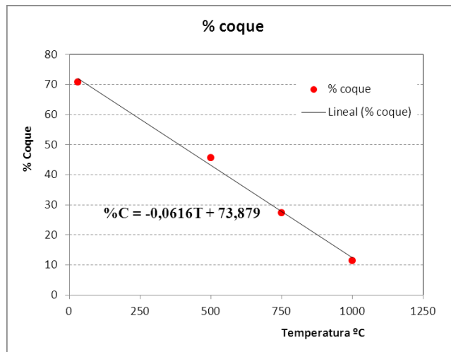
Figura 5. Modelo matemático lineal que relaciona el porcentaje de coque necesario en función de la temperatura para lograr la neutralización del lodo rojo, el cual se alcanza cuando el Ph es igual a 7.
