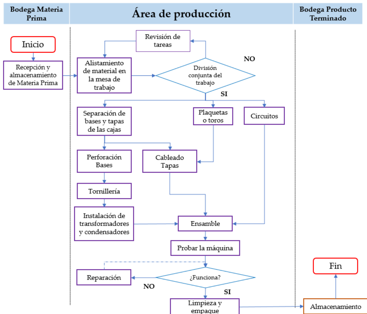
Figura. 3. Flujograma del proceso de producción de controles eléctricos de 40 K
