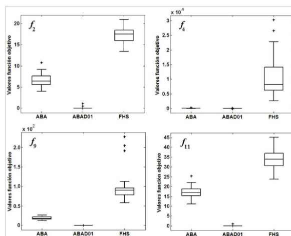
Figura 4: Diagramas de caja y bigotes para los resultados obtenidos sobre las instancias de problemas de optimización multimodal y no separable.
