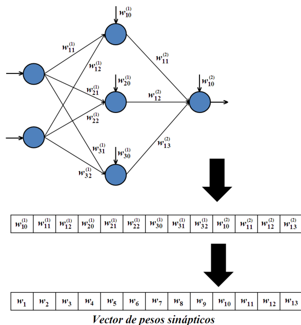
Figura 2: Representación de pesos sinápticos de una red hipotética de dos (02) capas.
